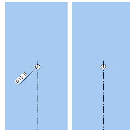
【notice 1. ガラス穴あけ寸法】
