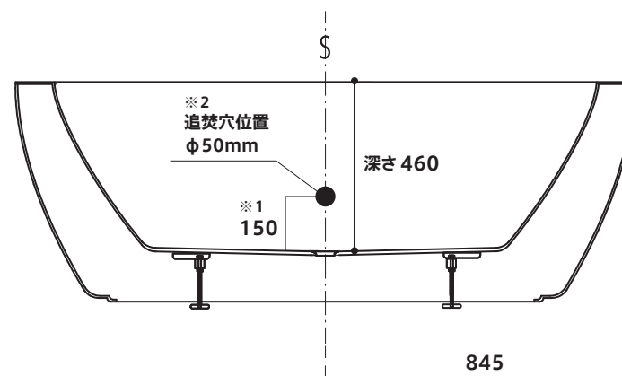
断面図
